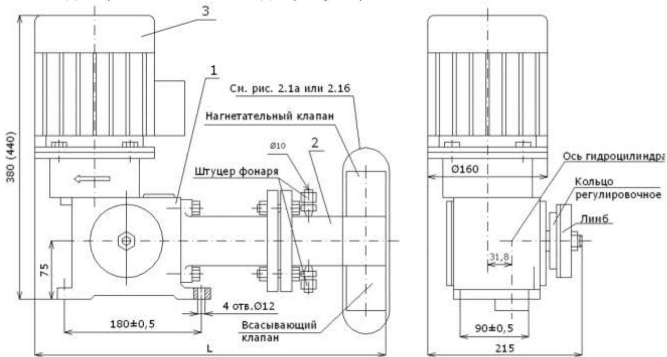
Рис. 1 - Дозировочный насос НД с редуктором АР30
